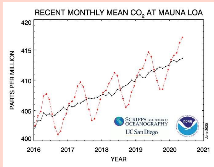
Les quatre dernières années à l'observatoire de Mauna Loa (Hawaï). En rouge, les données mensuelles avec une variabilité saisonnière. En noir, la tendance moyenne.
