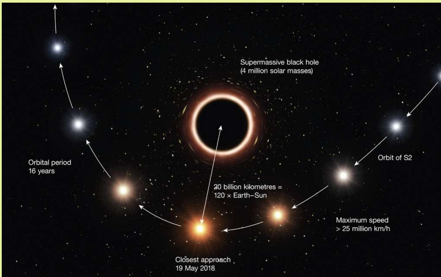
L'orbite elliptique de l'étoile S0-2 autour du trou noir supermassif au centre de la Voie lactée. © ESO, M. Kornmesser
